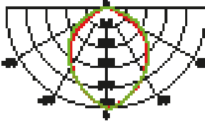
MIKROPRIISMATISKT BLÄNSKYDD
