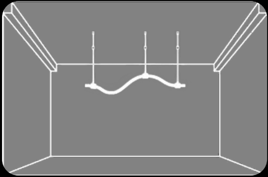
55263 Moonlight 360 pendelkit med plast clips.
