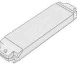
52162 75W / 24V DC (minsta belastning 20W) Mått: L=213 mm, B=54 mm, H=33 mm C10A = 10 st, C16A = 14 st
