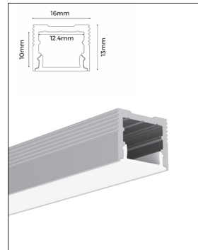
Aluminiumprofil-U 57002 Profillängd: 2500 mm Bredd: 16 mm Höjd: 13 mm Montageclips: 57102, 57103, 57104
