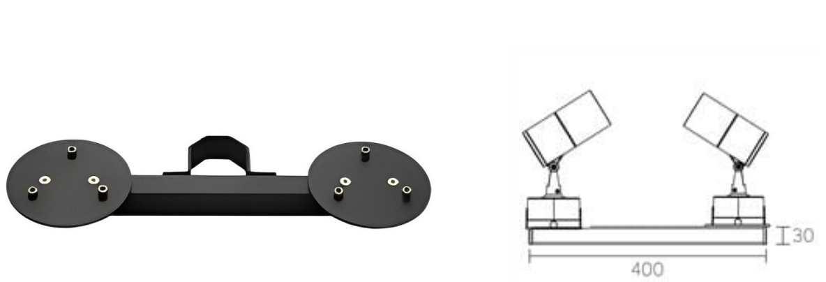
113053 Dubbelarm 2 x 25W Spirit, antracit
