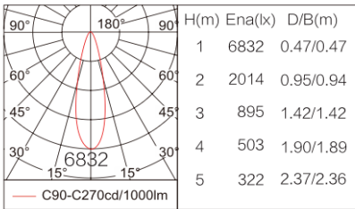
24° - 13W - 3000K - 90CRI
