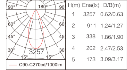
36° - 13W - 3000K - 90CRI
