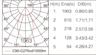
50° - 13W - 3000K - 90CRI
