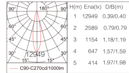
15° - 13W - 3000K - 90CRI
