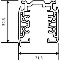
Global trac pro Tänd/släck, Fasdim, Casambi
